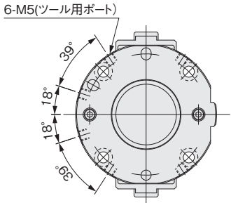
配管寸法図
