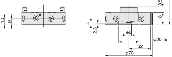
取付寸法図
