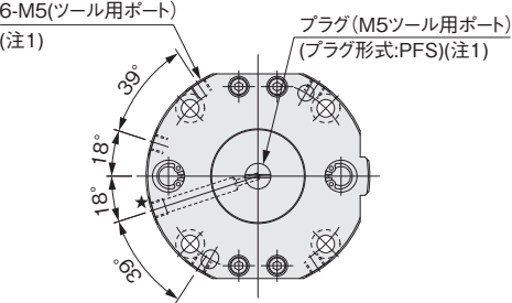
配管寸法図
