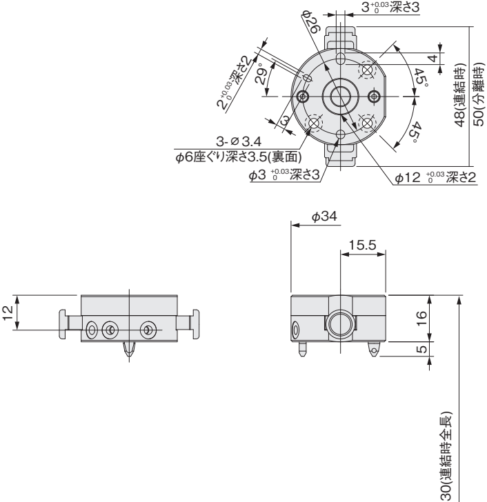
取付寸法図
