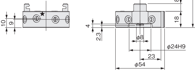
取付寸法図
