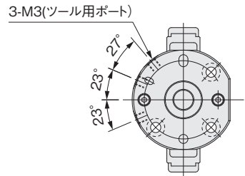
配管寸法図
