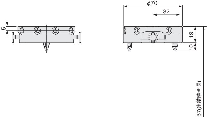
取付寸法図
