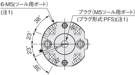
配管寸法図
