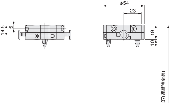
取付寸法図
