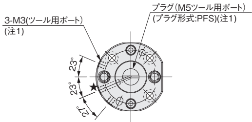
配管寸法図
