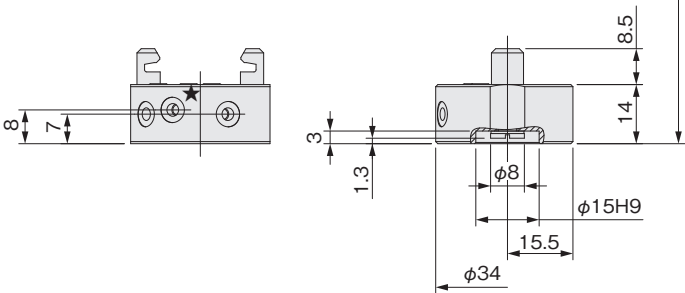
取付寸法図
